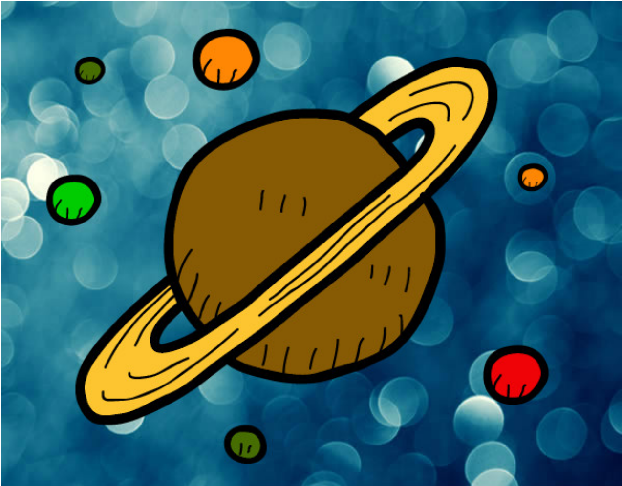
Satélites de Saturno pintado por valeria21
