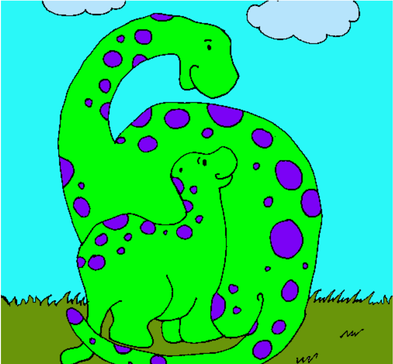
Dinosaurios pintado por loy3
