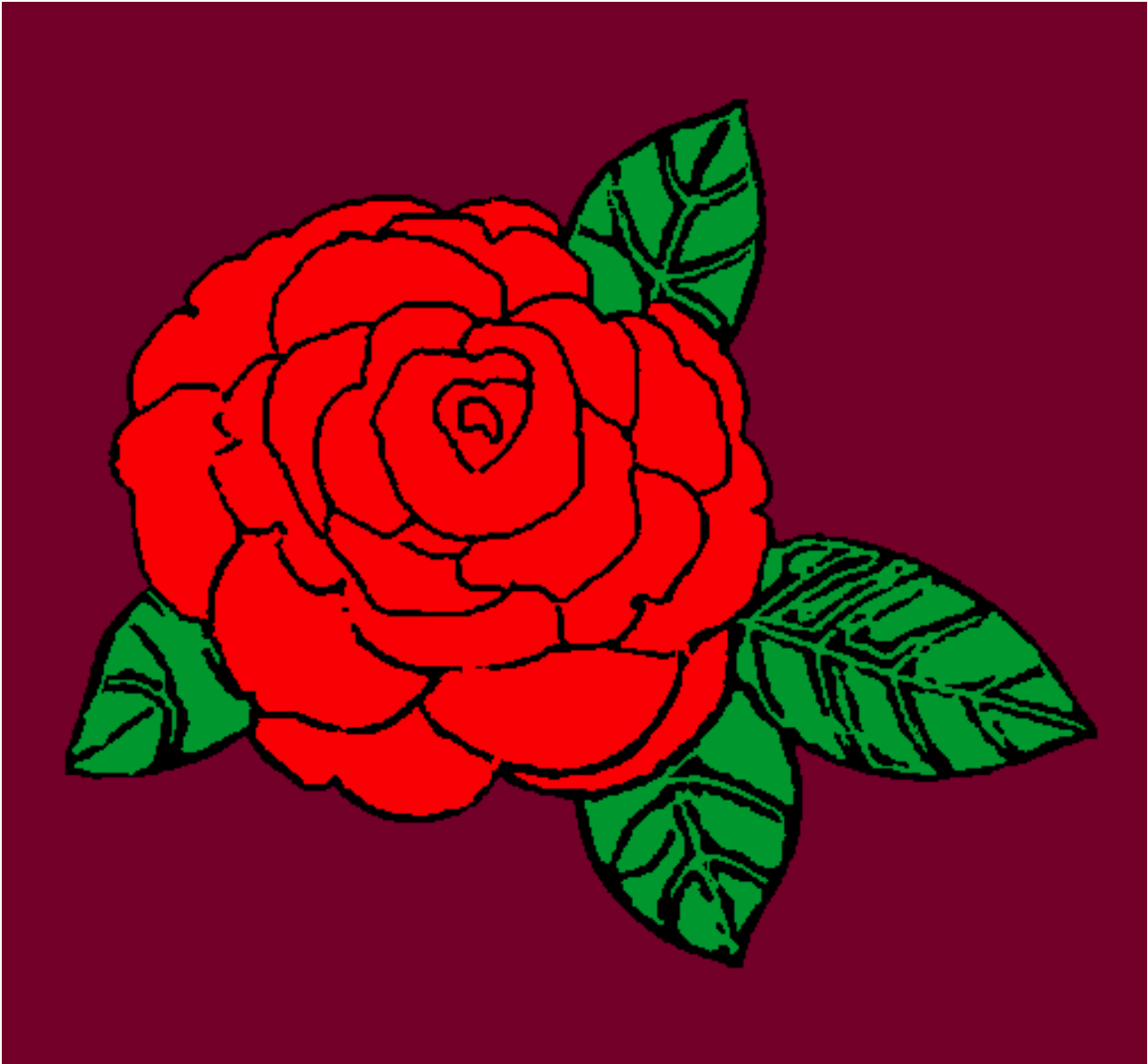
Rosa pintado por albita
