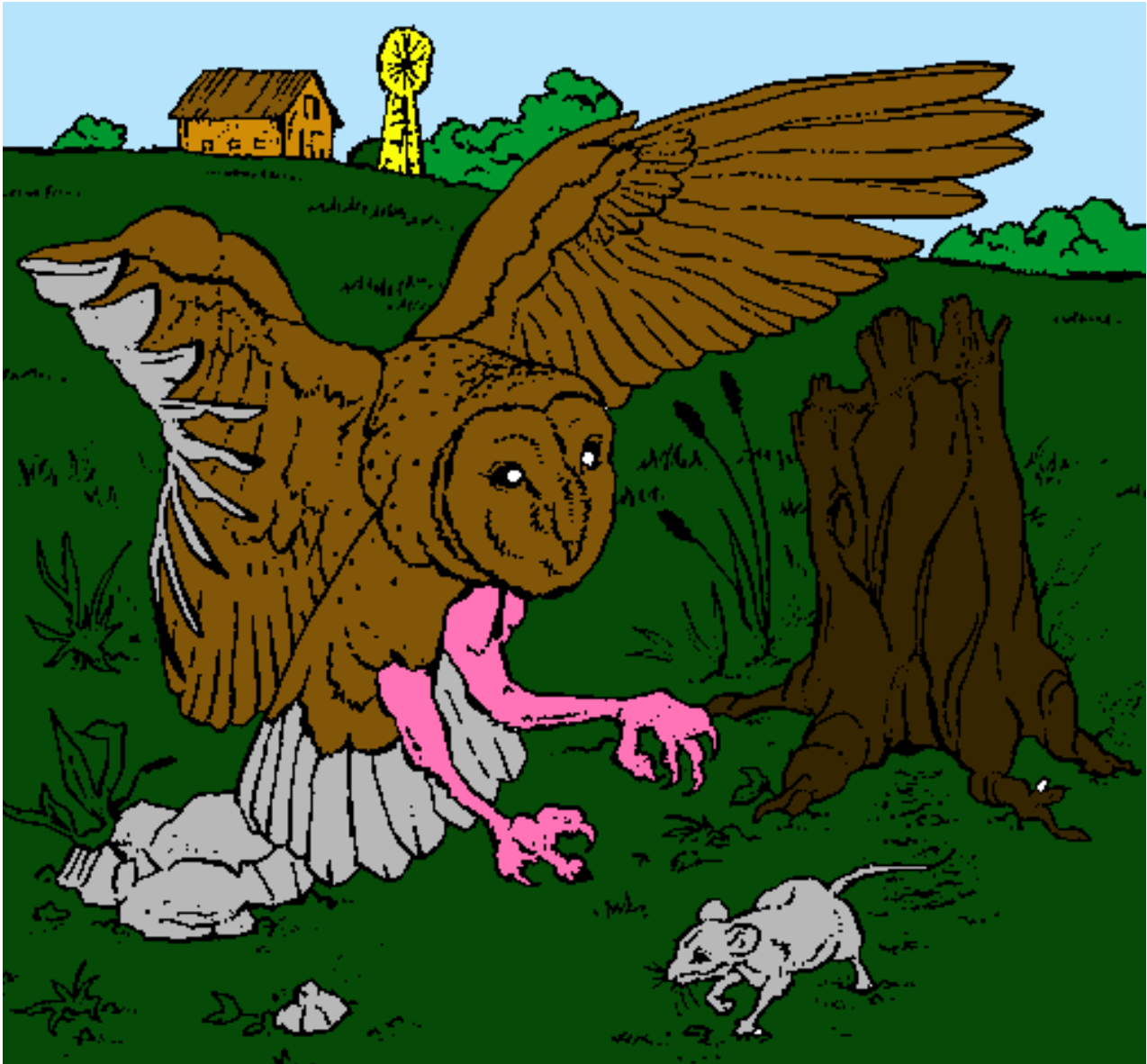
Búho cazando pintado por 43221nugy777
